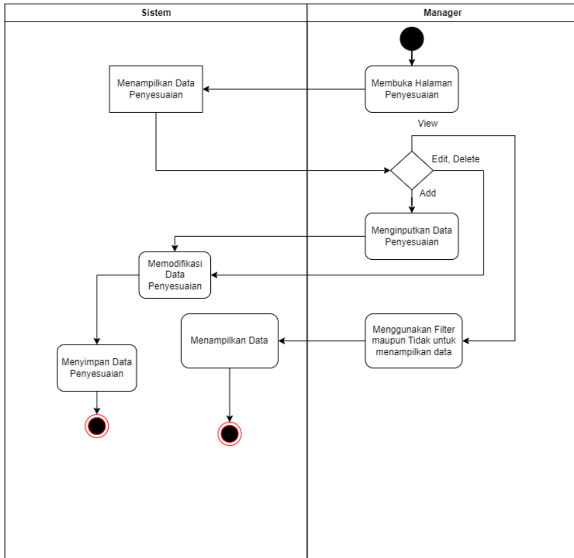
Gambar 3.13 Activity Diagram Penyesuaian
