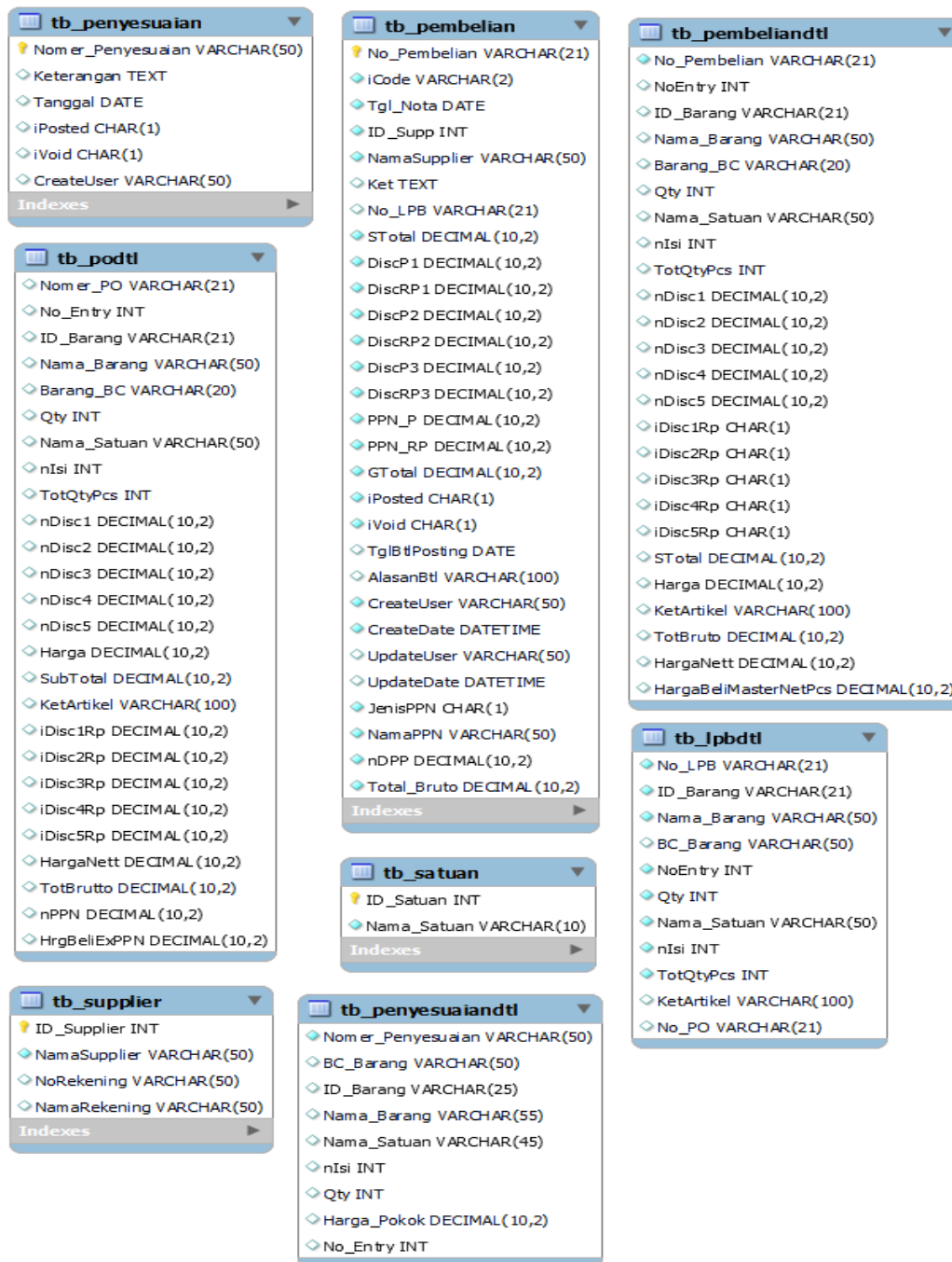
Gambar 3.37 Design Sistem Keseluruhan bagian 2
