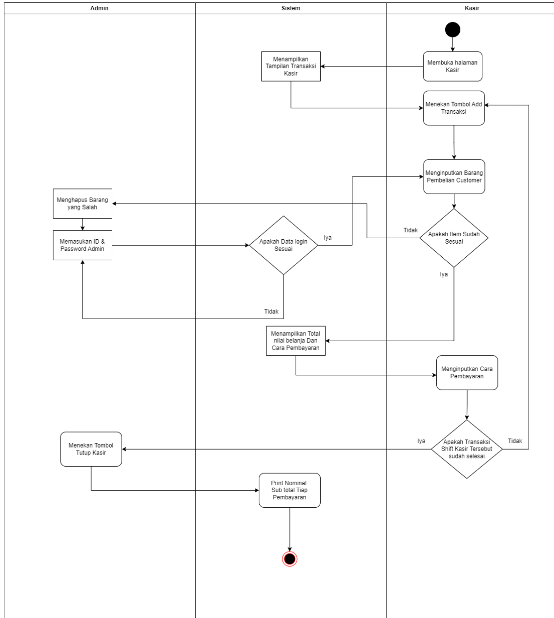
Gambar 3.11 Activity Diagram Penjualan Kasir
